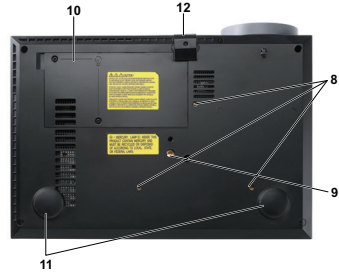
底視圖
